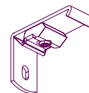
ESCUADRA CON CLIK 35 MM T 60 MM
